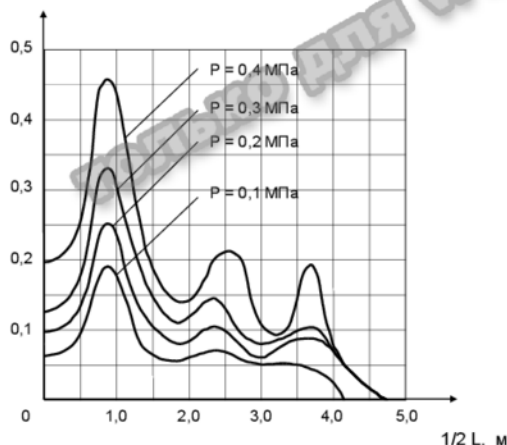
Рис. 2. Эпюры удельного расхода, Ду 8 мм.
