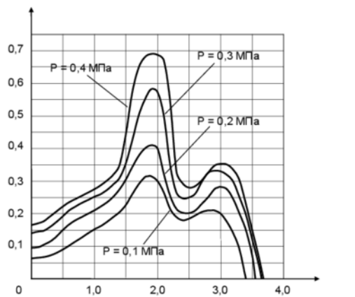
Рис. 3. Эпюры удельного расхода, Ду 12 мм. 1/2 L, м
