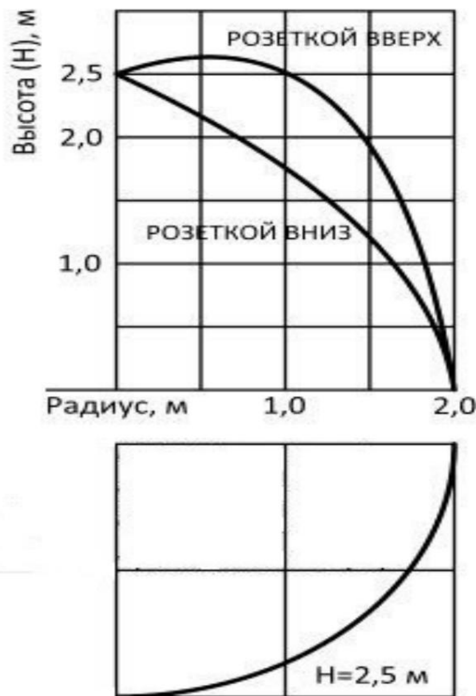
Эпюры орошения водой (пенной)
