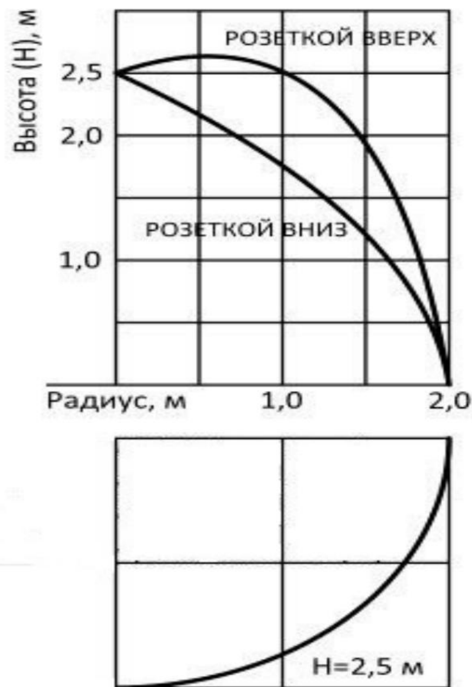
Эпюры орошения водой (пеной)
